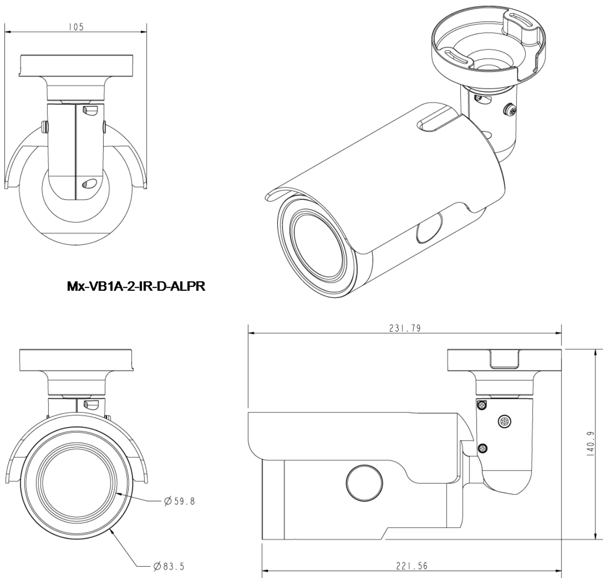
Fig. 2 : 2MP Vandal Bullet ALPR Camera: Toutes les mesures sont en mm
