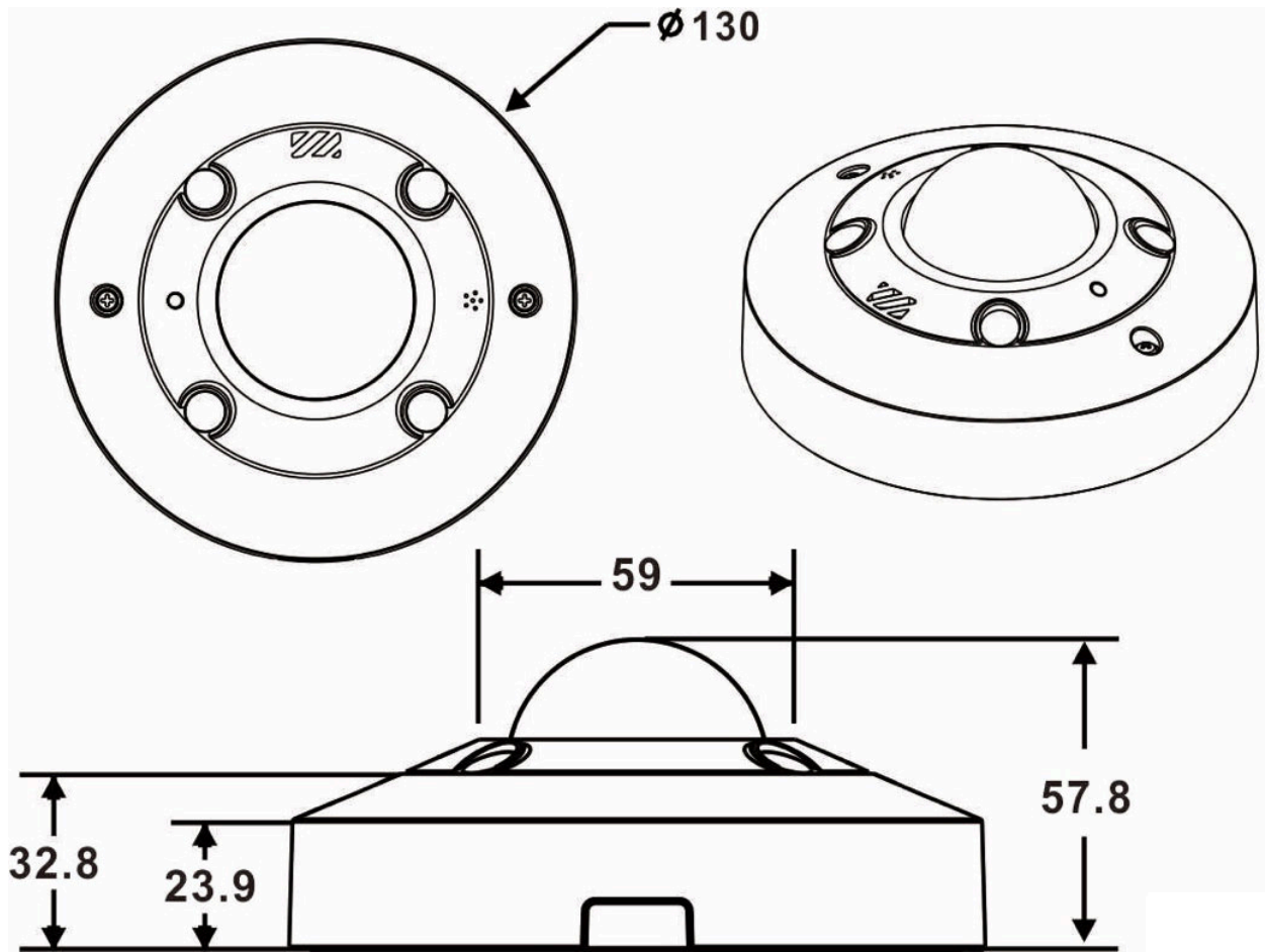
Fig. 1: 12MP Vandal Hemispheric Analytics Indoor Camera: Tutte le misure sono espresse in mm
