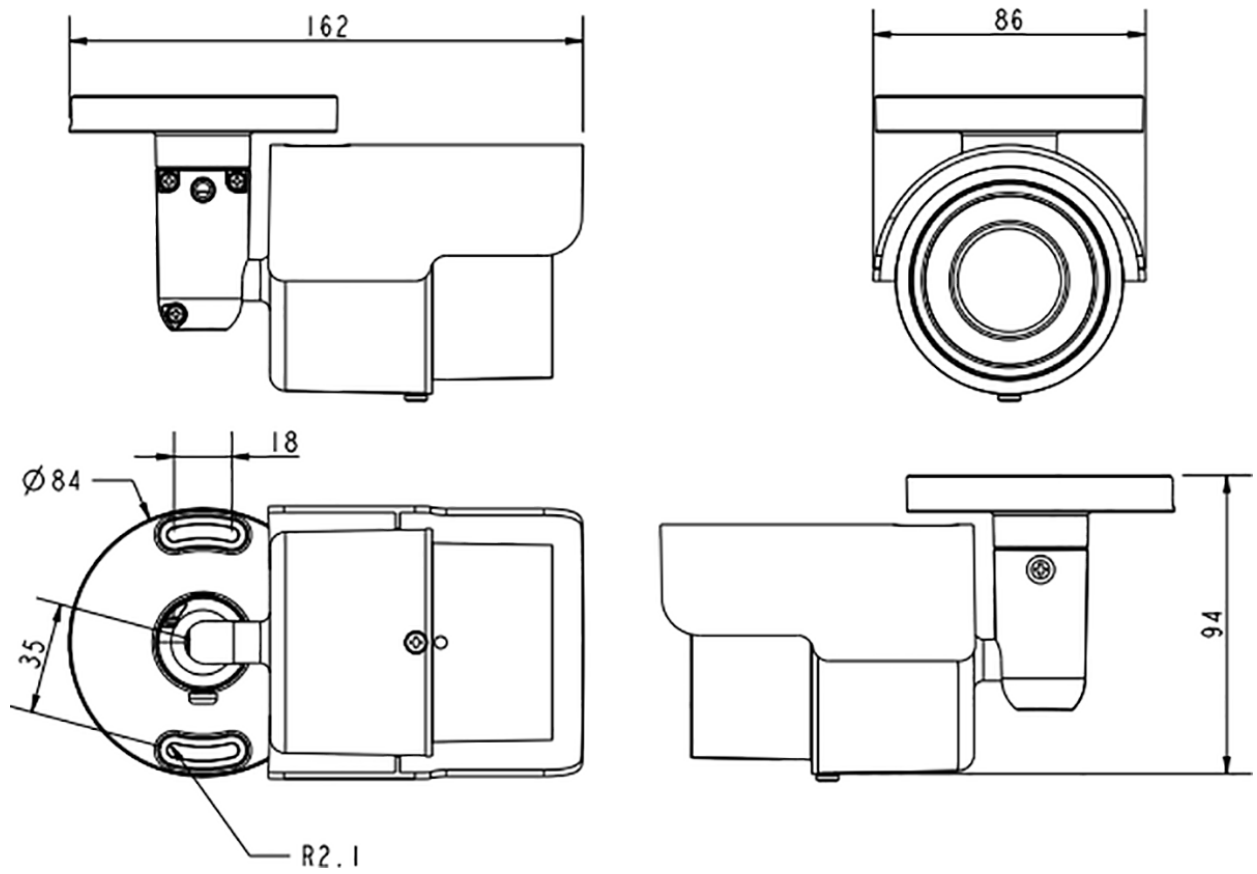
Abb. 1: Mx-BC2A-2-IR: Alle Maße in mm
