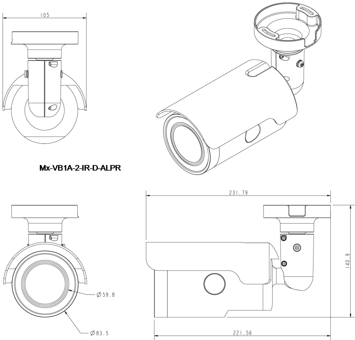
Abb. 2: Mx-VB1A-2-IR-D-ALPR: Alle Maße in mm
