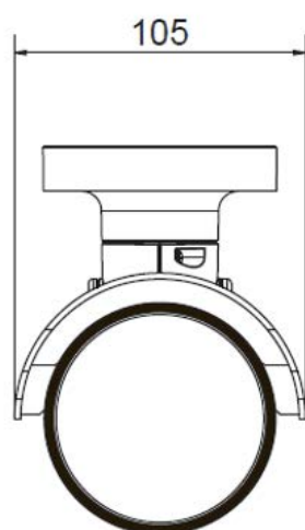
Abb. 1: Mx-VB1A-8-IR-VA: Alle Maße in mm
