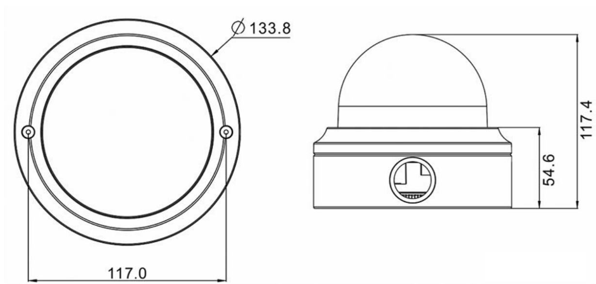
Fig. 1: Mx-VD2A-5-IR-VA: Todas las medidas en mm
