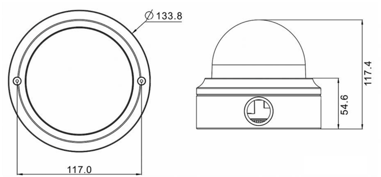
Abb. 1: Mx-VD3A-2-IR-VA: Alle Maße in mm
