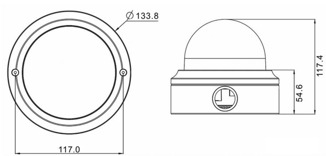
Abb. 1: Mx-VD1A-8-IR-VA: Alle Maße in mm
