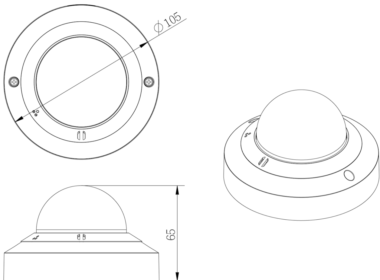
Fig. 1: Mx-MD1A-5-IR: Todas las medidas en mm
