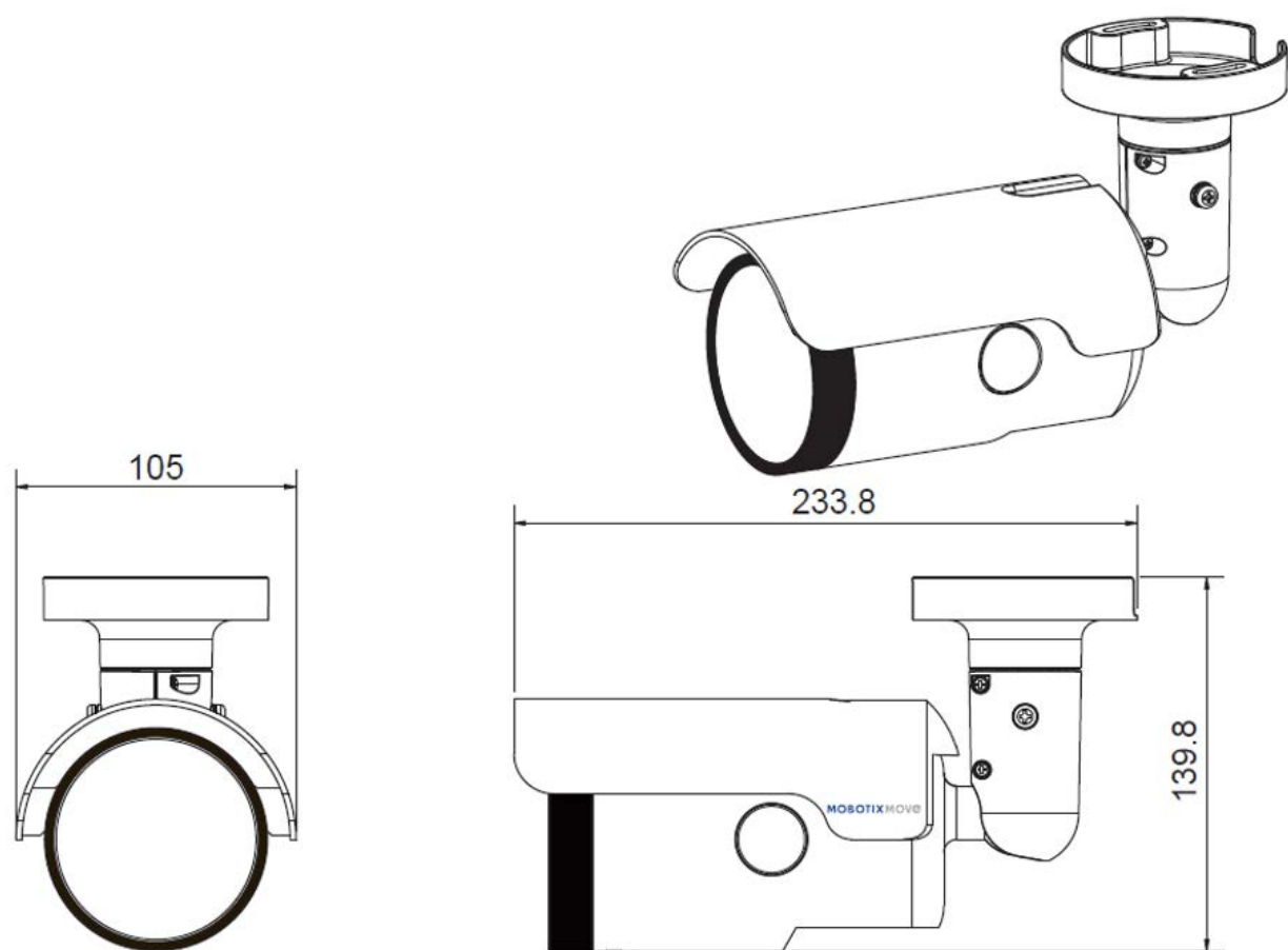
Fig. 1: Mx-VB1A-8-IR-VA: Todas las medidas en mm
