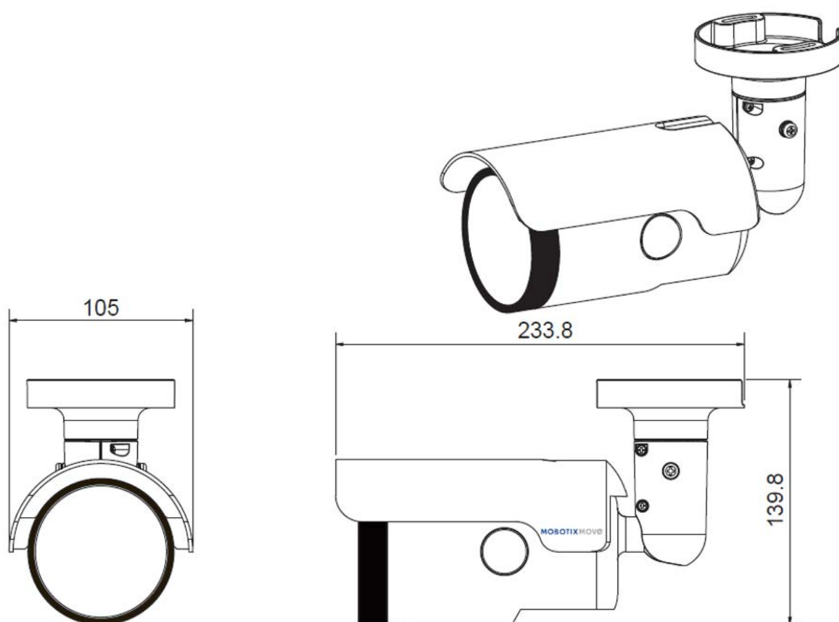
Abb. 1: Mx-VB3A-2-IR-VA: Alle Maße in mm
