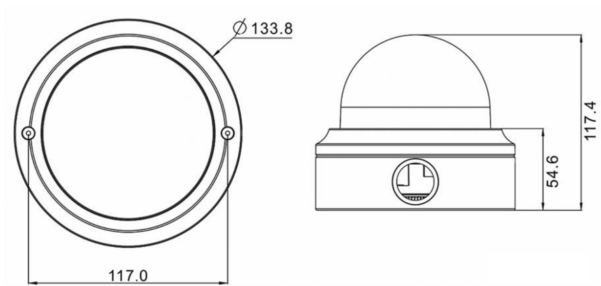
Fig. 1 : Mx-VD1A-8-IR-VA: Toutes les mesures sont en mm
