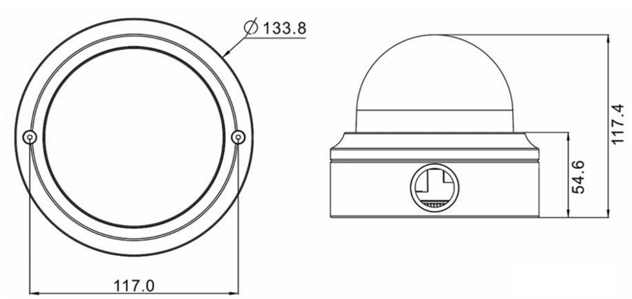
Abb. 1: Mx-VD2A-5-IR-VA: Alle Maße in mm
