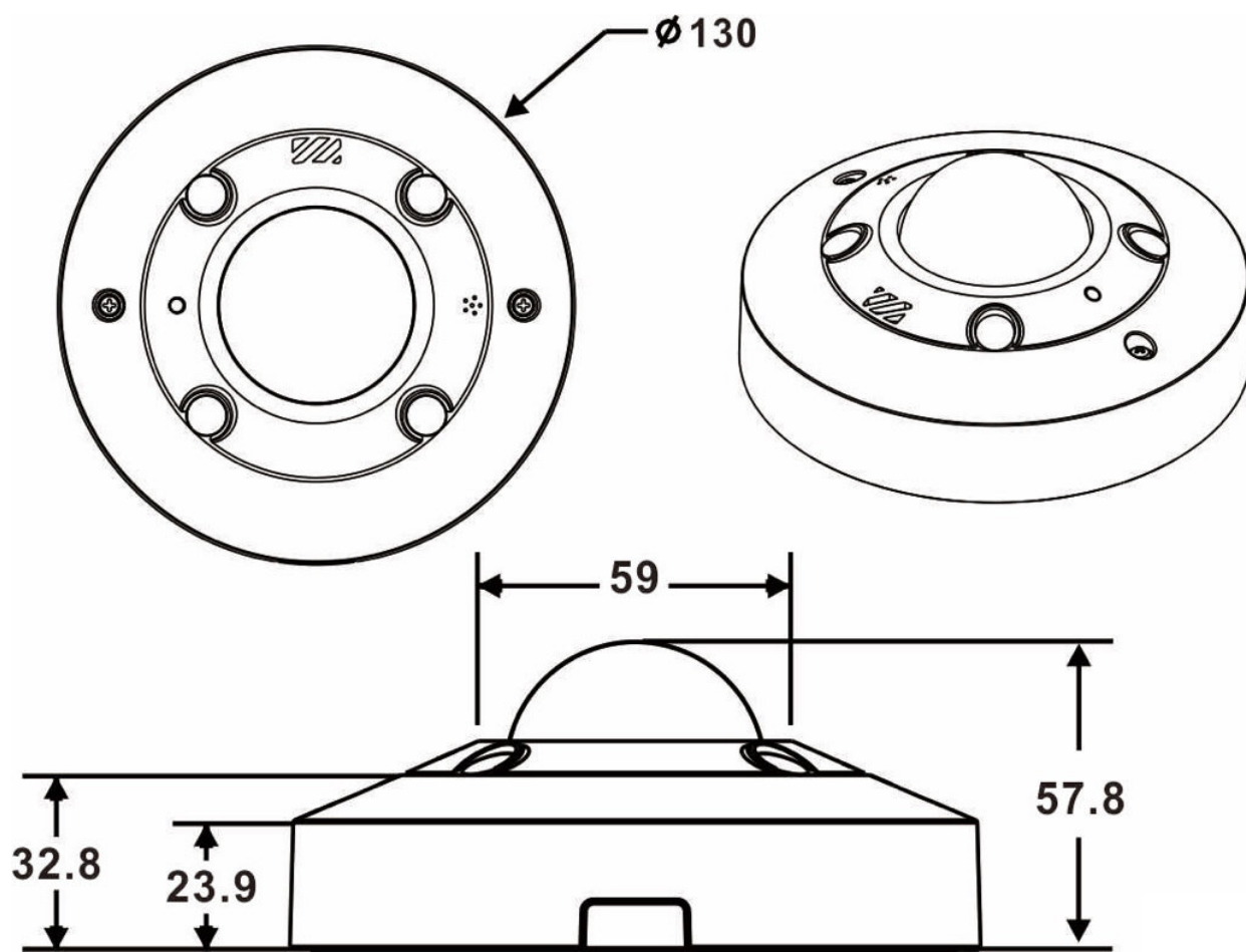
Fig. 1 : Mx-VH1A-12-IR-VA: Toutes les mesures sont en mm
