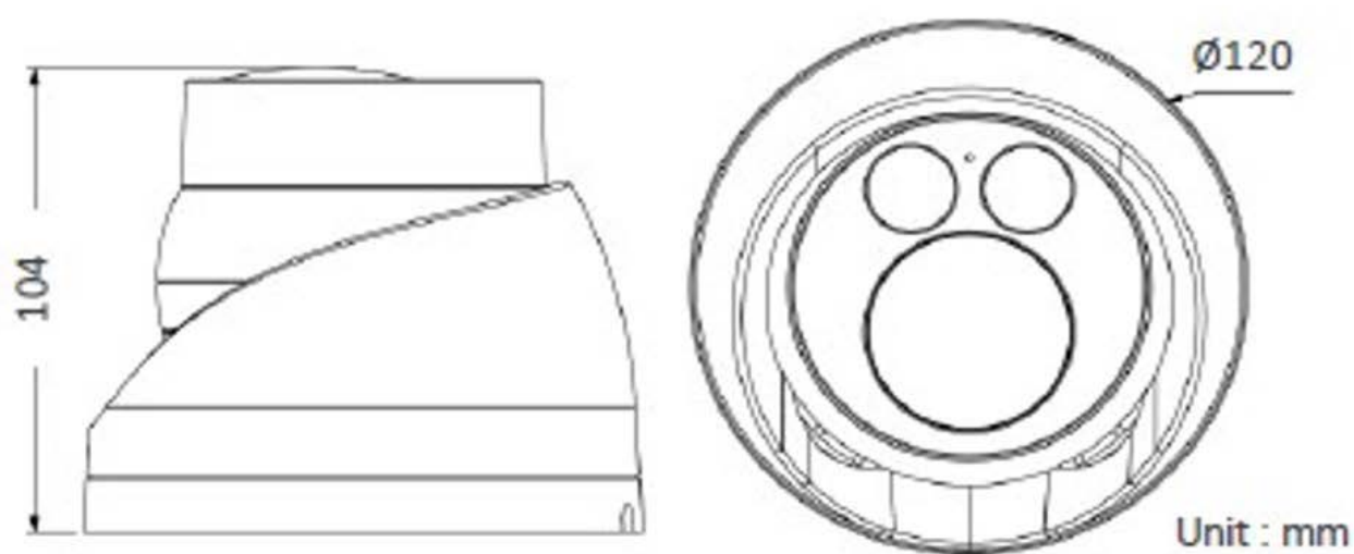
Fig. 1 : Mx-VT1A-503-IR: Toutes les mesures sont en mm
