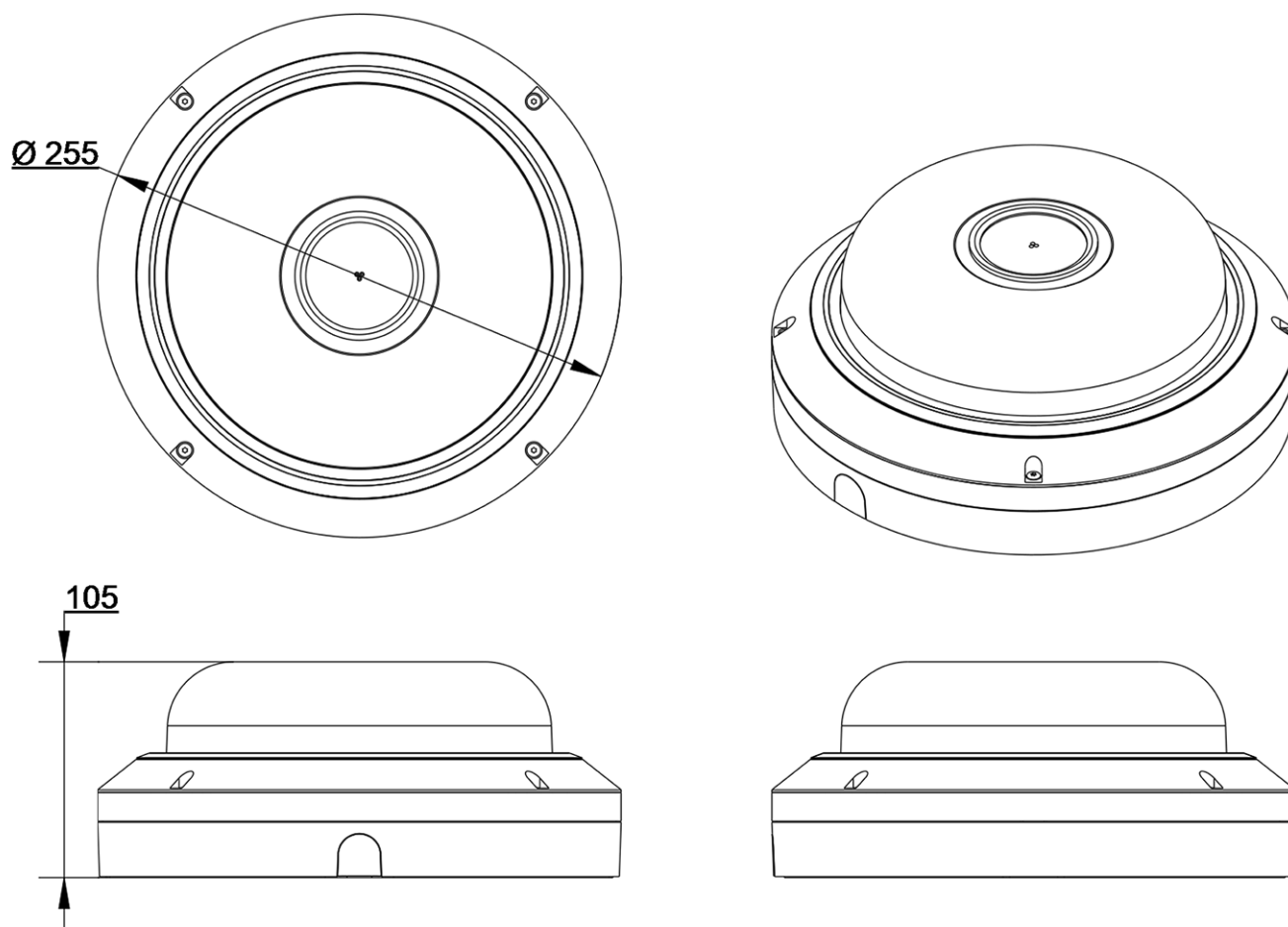
Fig. 1 : Mx-VM1A-20-IR-VA: Toutes les mesures sont en mm
