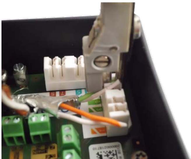
Abb. 27: Mit dem LSA+/Krone-Tool angeschlossene Netzwerkdrähte
