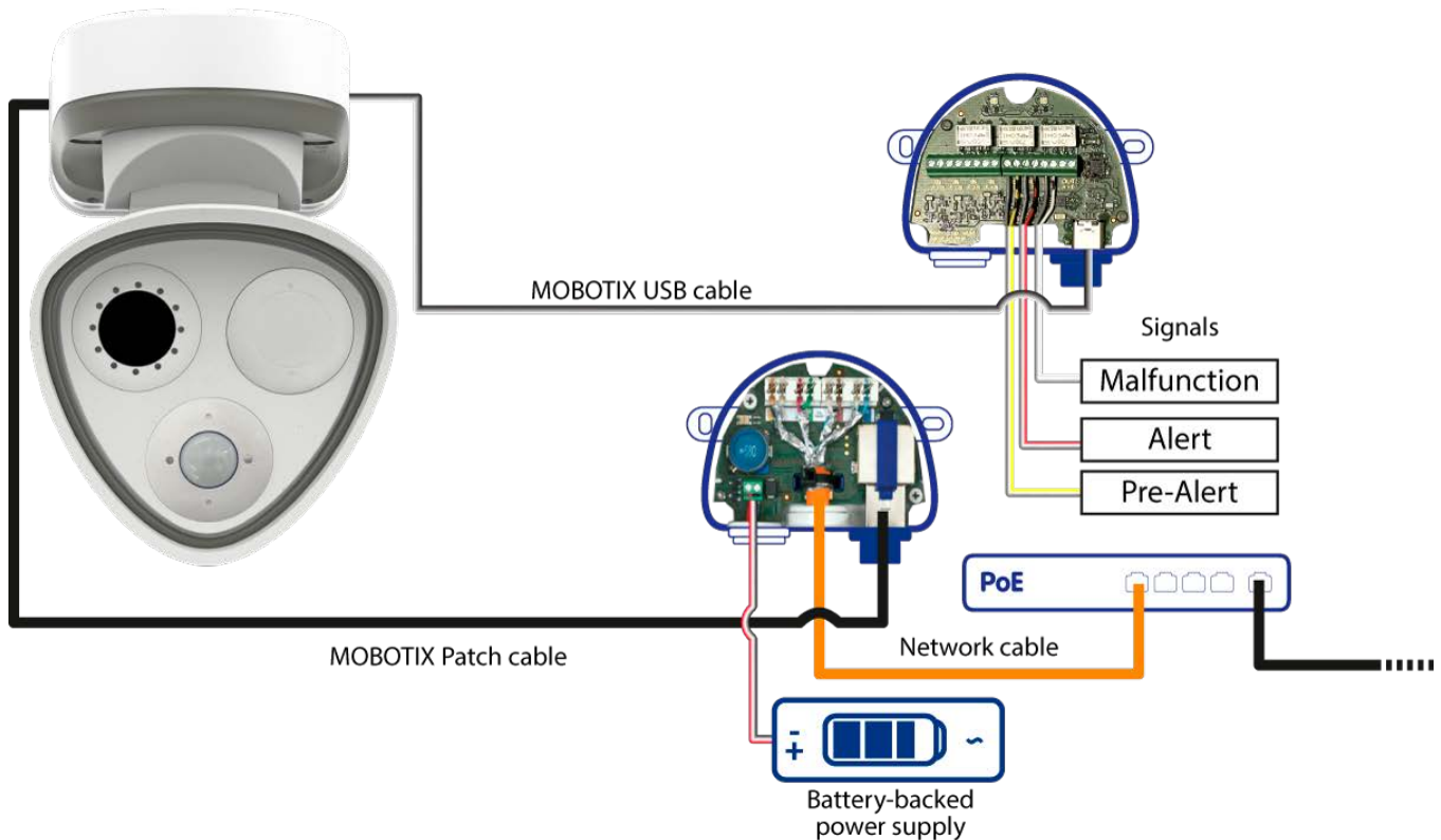
Abb. 2: Verdrahtung der M73 EN54 Bundle-V2
