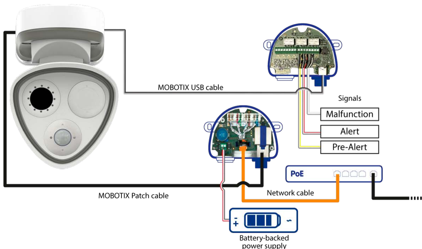
Fig. 2: Cableado del M73 EN54 Bundle-V2
