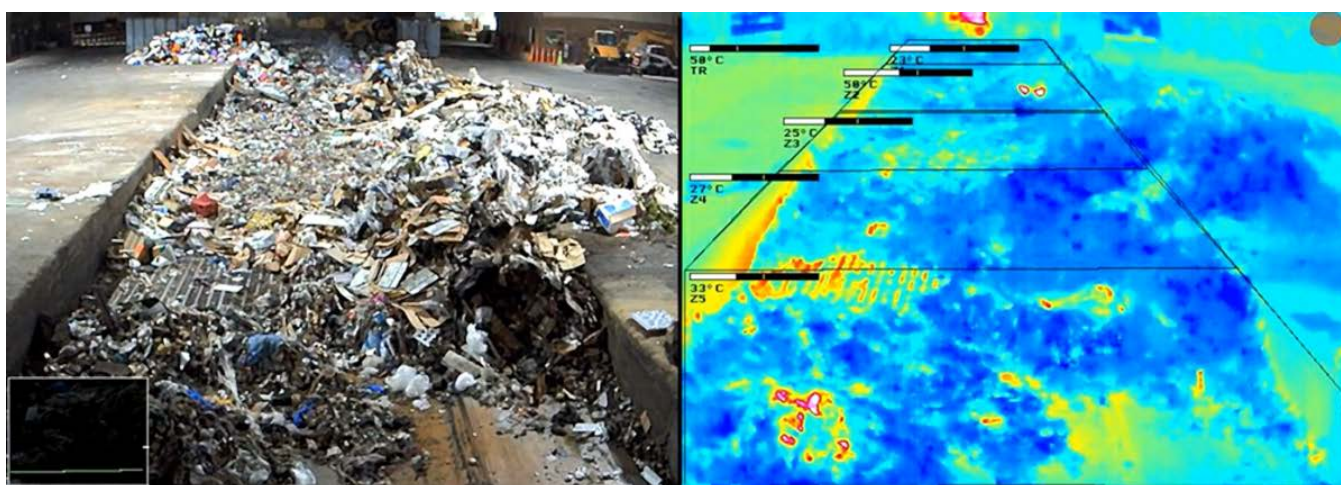
Fig. 3: RTI come misura preventiva in un impianto di riciclaggio utilizzando aree di misura impilate con compensazione individuale della distanza per una misurazione accurata.
