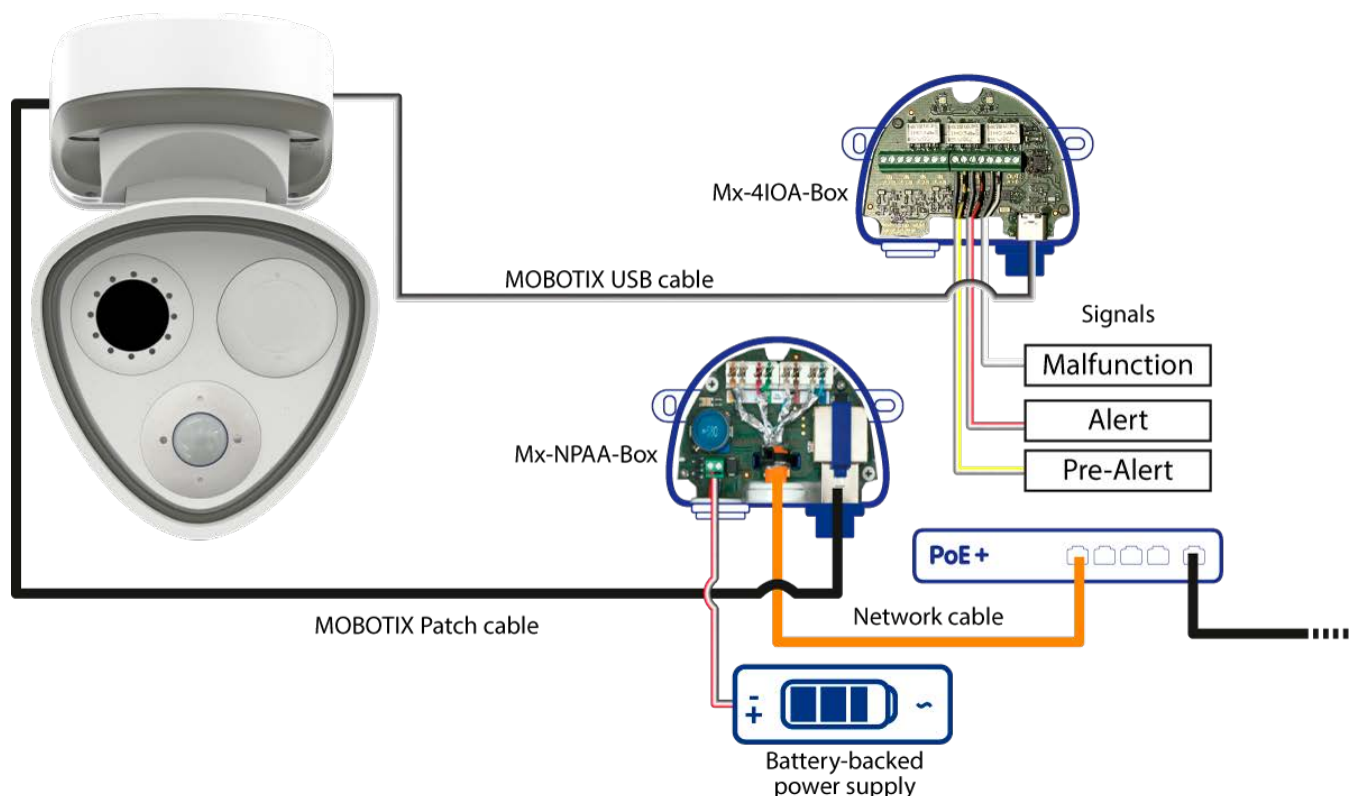
Fig. 2 : Câblage de la M73 EN54 Bundle-V2
