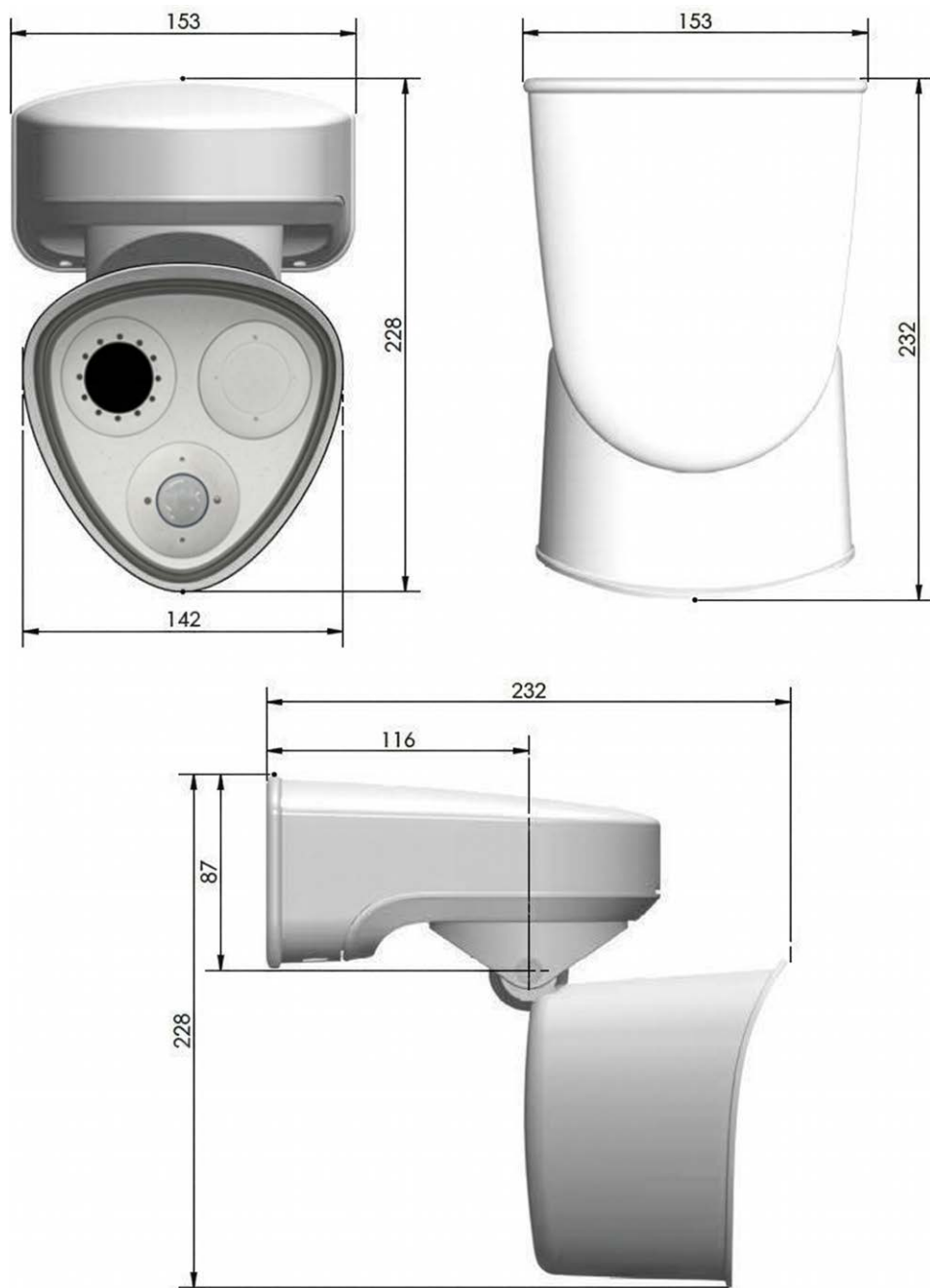
Fig. 10 : MOBOTIX M73: Toutes les mesures sont en mm
