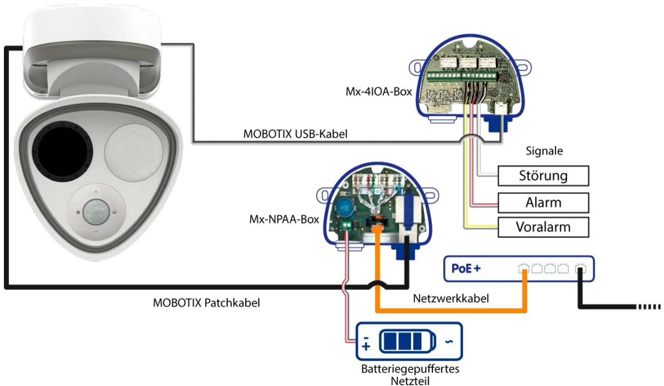
Abb. 2: Verdrahtung der M73 EN54 Bundle-V3
