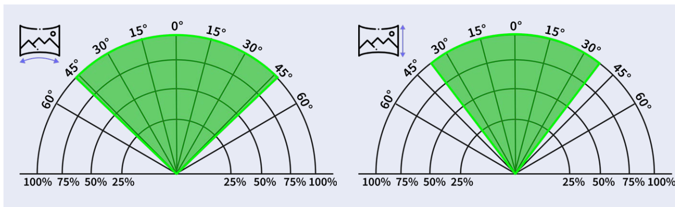
Objetivo con ángulo de visión horizontal de 95
