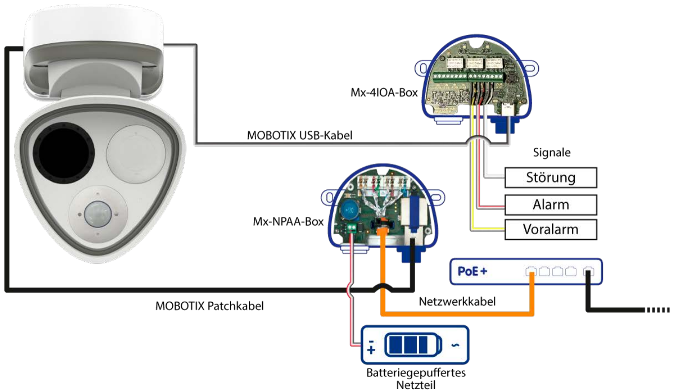
Abb. 5: Verdrahtung der M73 FM Bundle
