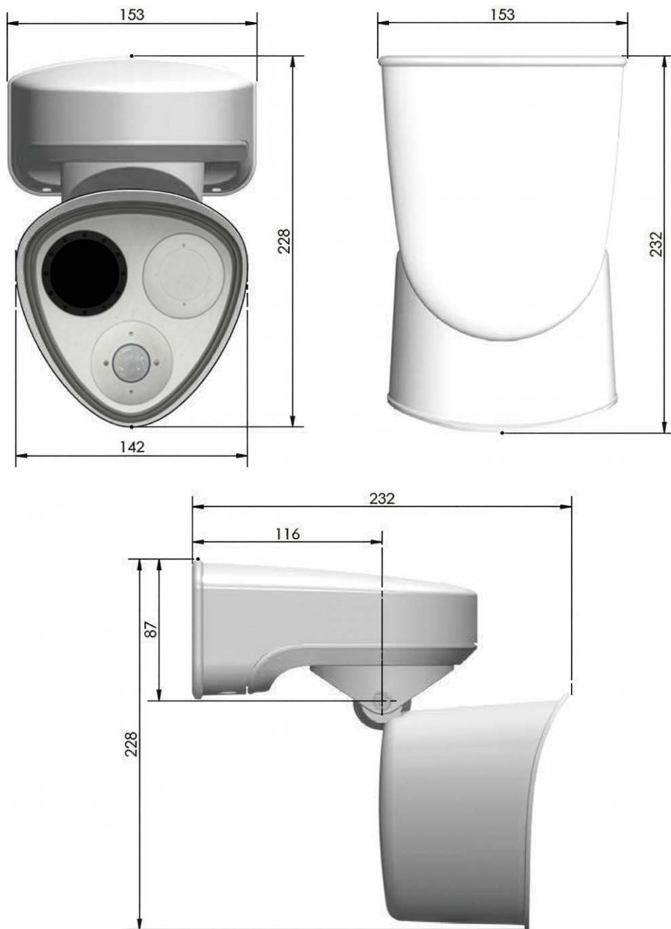
Abb. 13: MOBOTIX M73: Alle Abmessungen in mm
