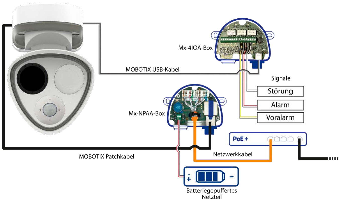
Abb. 5: Verdrahtung der M73 FM Bundle
