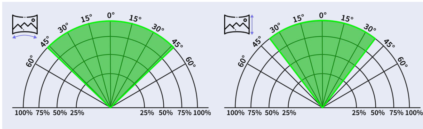
Gris: campo de visión; verde: zona de detección de llama
