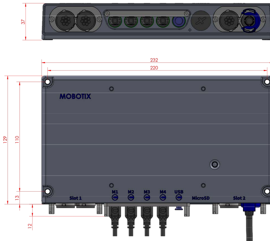
Fig. 9: MOBOTIX M73: Todas las medidas en mm
