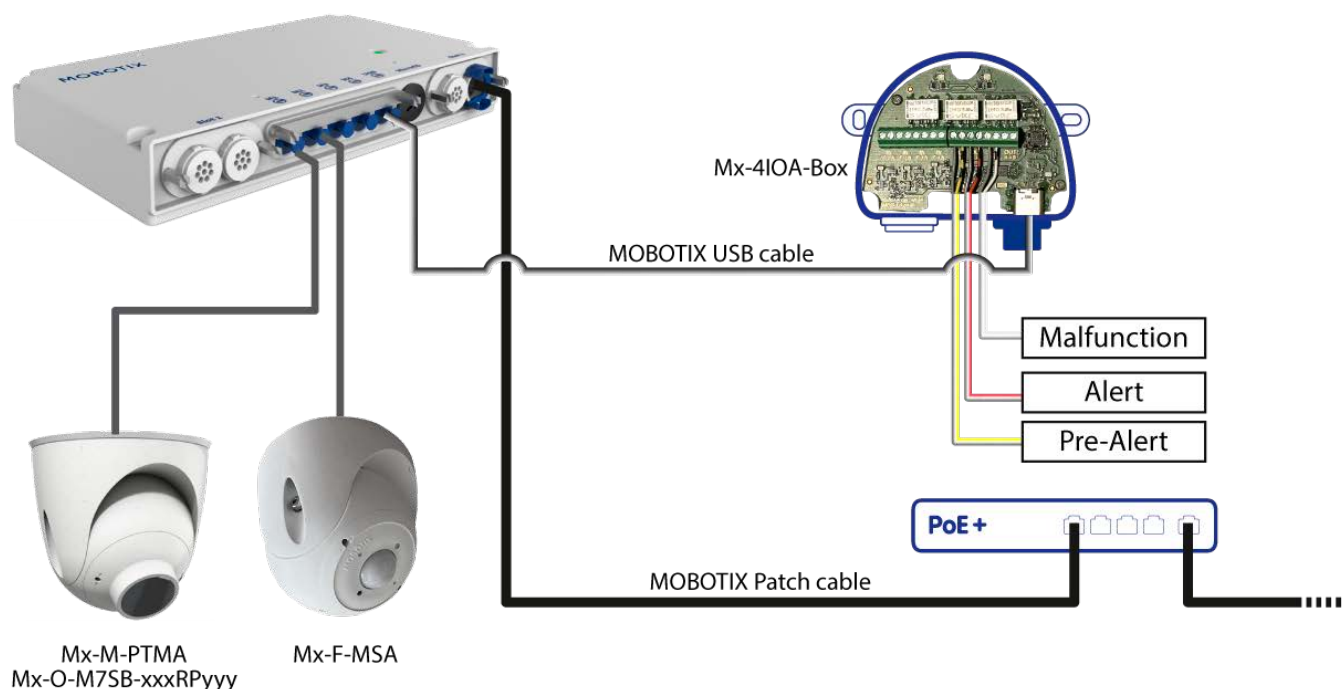
Fig. 1: Cableado del S74 EN54 Bundle-V2
