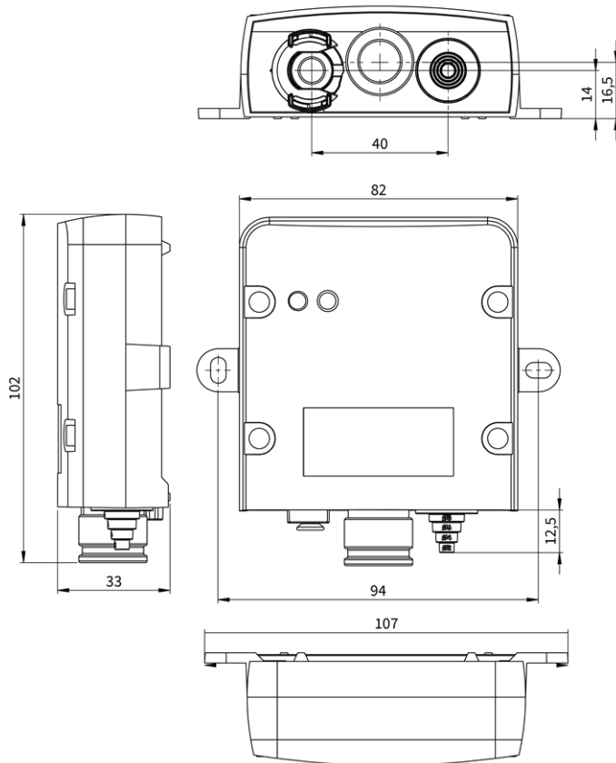
Abb. 2: MOBOTIX M73: Alle Abmessungen in mm
