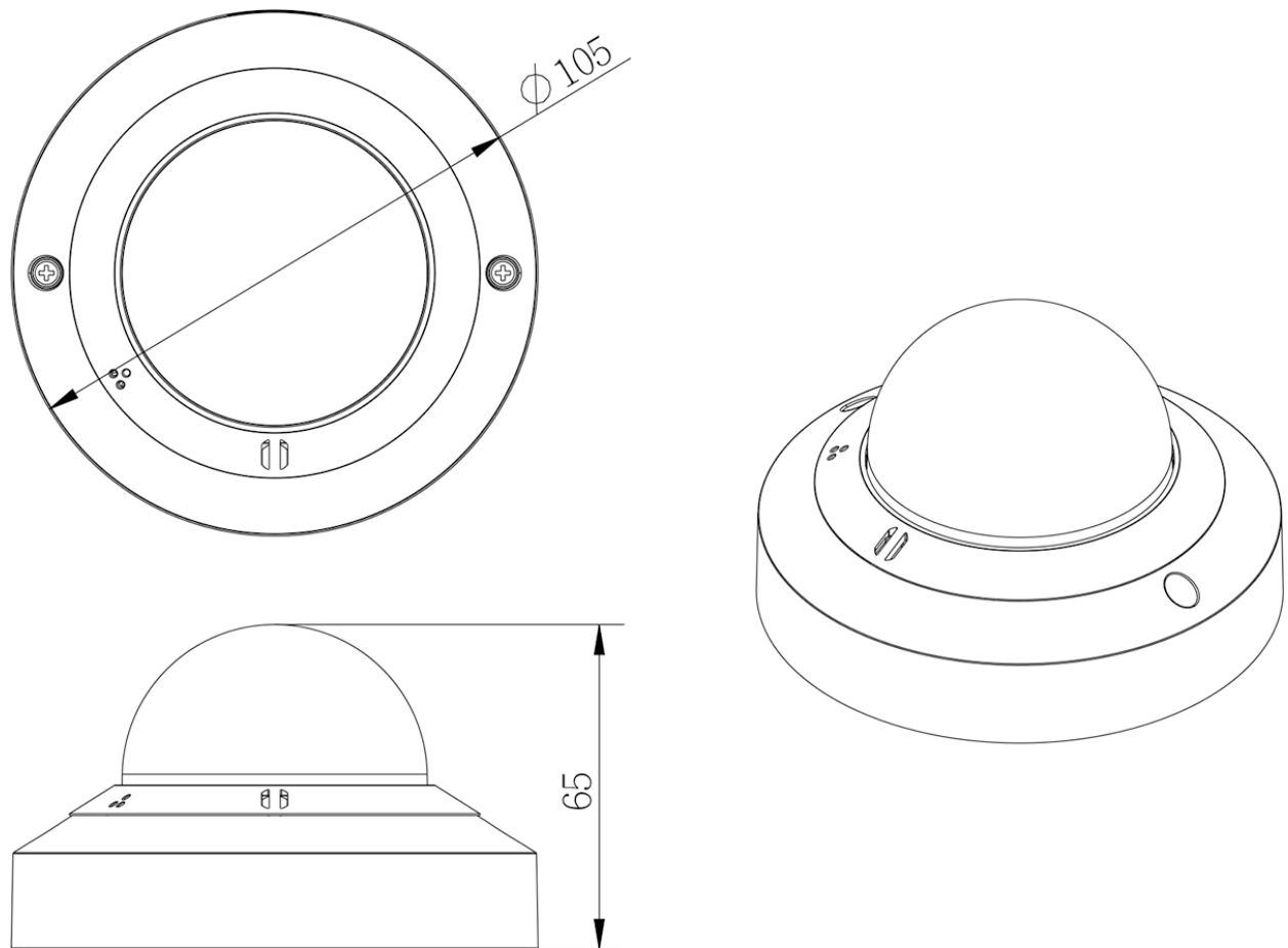
Abb. 1: Mx-MD1A-5-IR: Alle Abmessungen in mm
