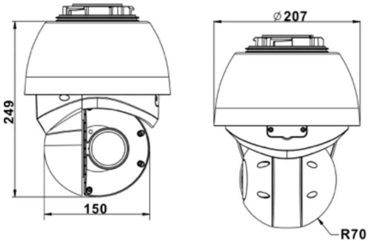
Abb. 1: Mx-SD1A-540-IR-VA: Alle Abmessungen in mm
