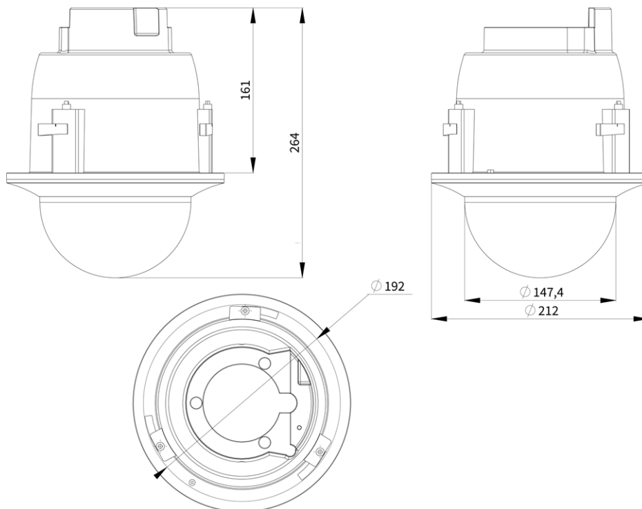
Abb. 1: Mx-SD2A-230-LL-FM-VA: Alle Abmessungen in mm
