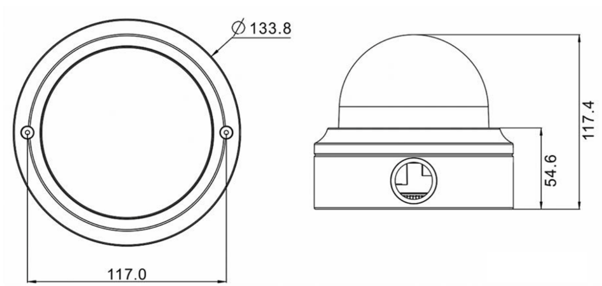
Fig. 1: Mx-VD1A-8-IR-VA: Todas las medidas en mm
