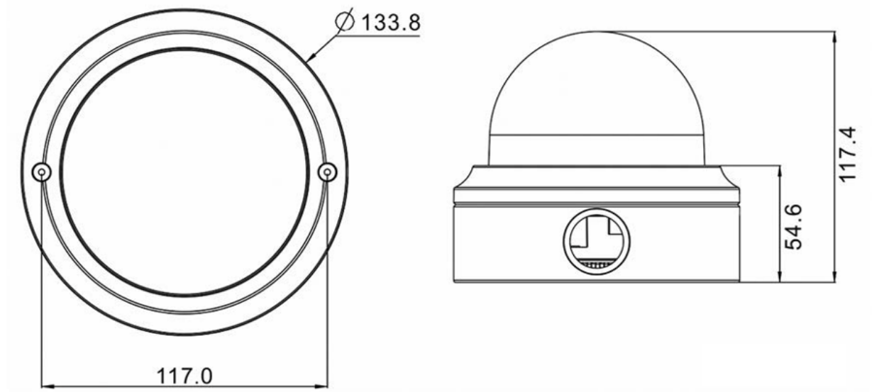
Abb. 1: Mx-VD2A-2-IR: Alle Abmessungen in mm
