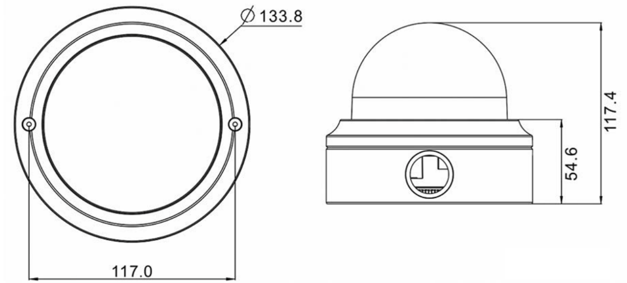
Fig. 1: Mx-VD2A-2-IR: Todas las medidas en mm
