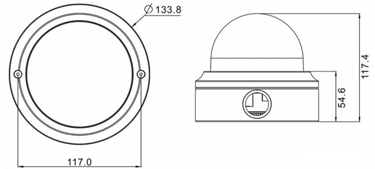
Fig. 1 : Mx-VD2A-2-IR: Toutes les mesures sont en mm
