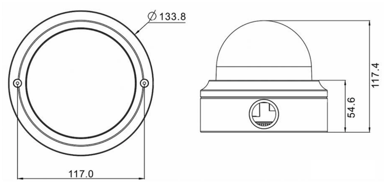
Abb. 1: Mx-VD3A-2-IR-VA: Alle Abmessungen in mm
