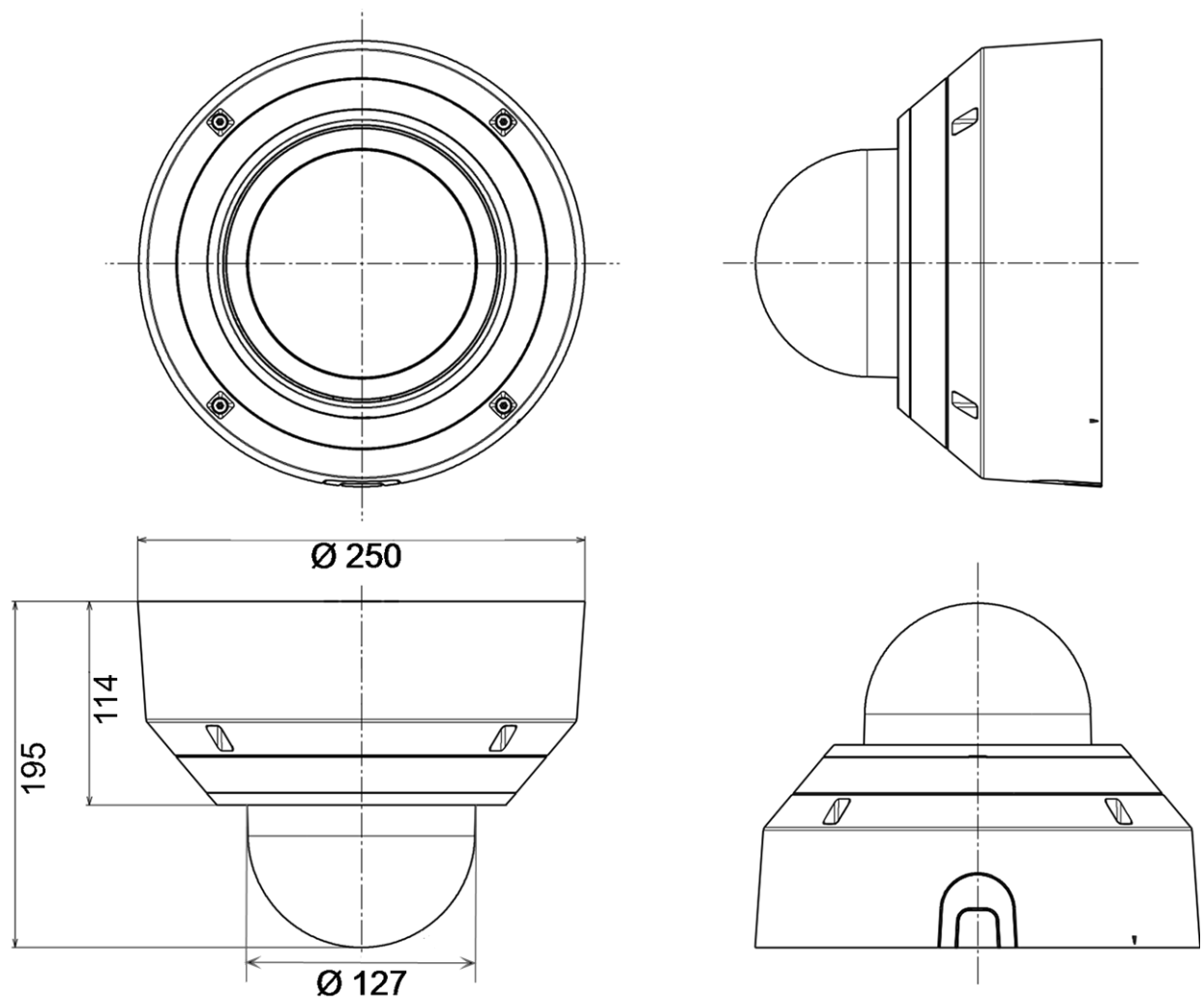
Abb. 1: Mx-VMSD1A-2021-VA: Alle Abmessungen in mm
