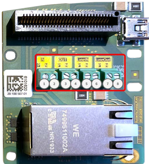
Terminal-Anschlüsse Anschlussdose RJ45
