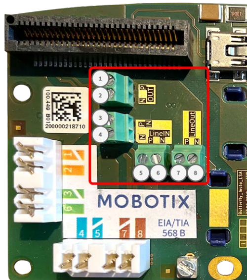
Terminal-Anschlüsse Anschlussdose LSA
