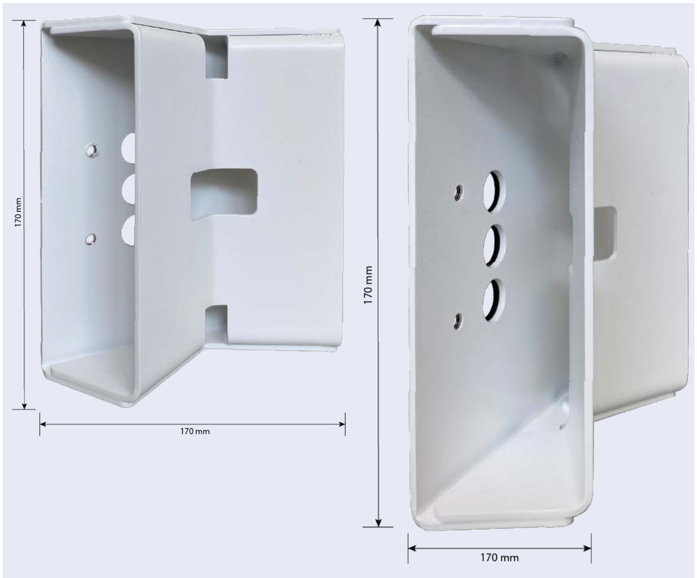
Abb. 8: Abmessungen M73 Masthalterung - Rückansicht
