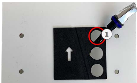
Abb. 10: Vorbereitet für Anschlussdose RJ45
