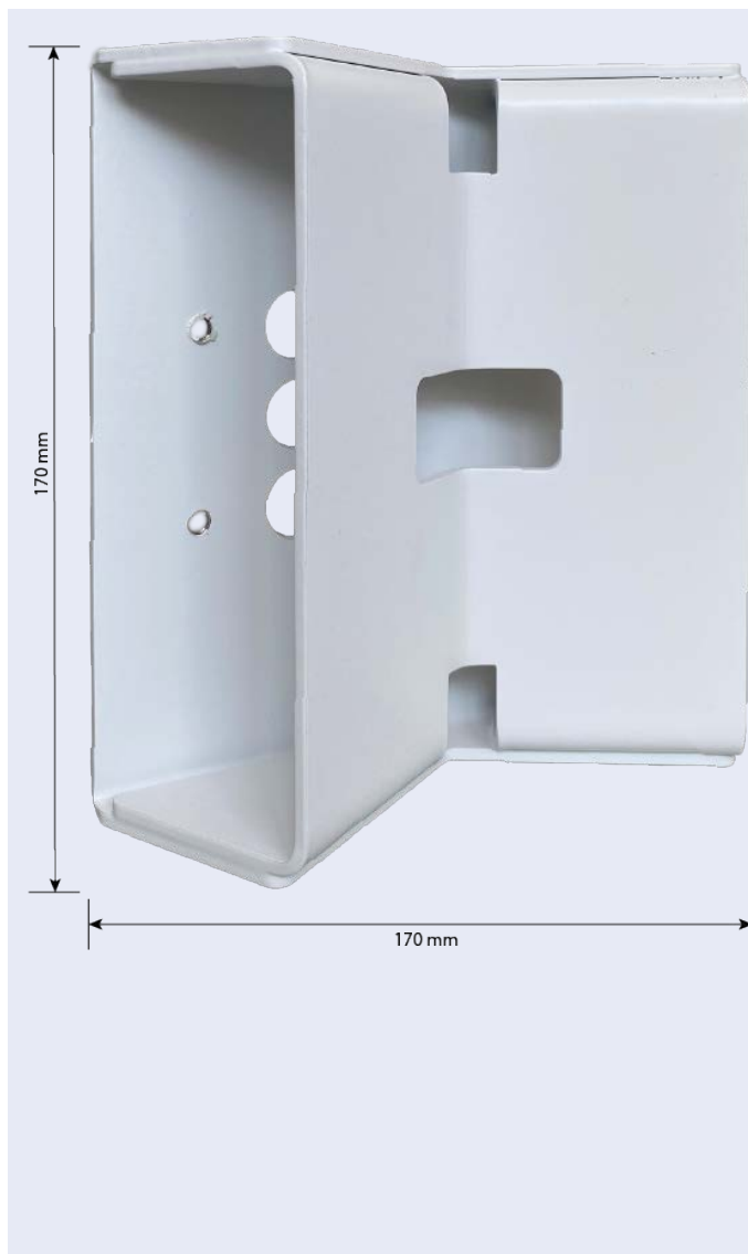
Fig. 8: Dimensiones M73 montaje en poste - vista trasera
