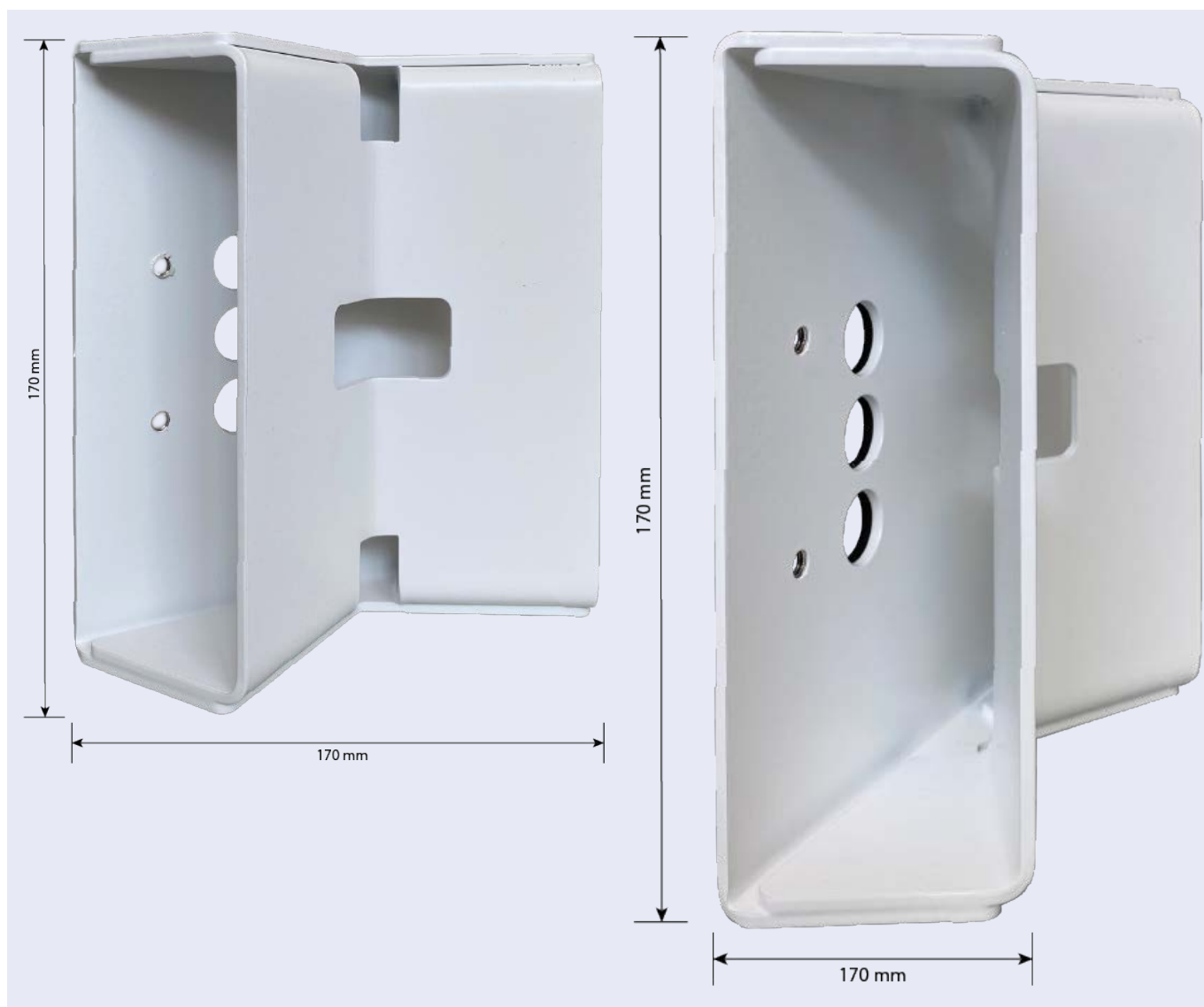
Fig. 8 : Dimensions M73 montage sur poteau - vue arrière
