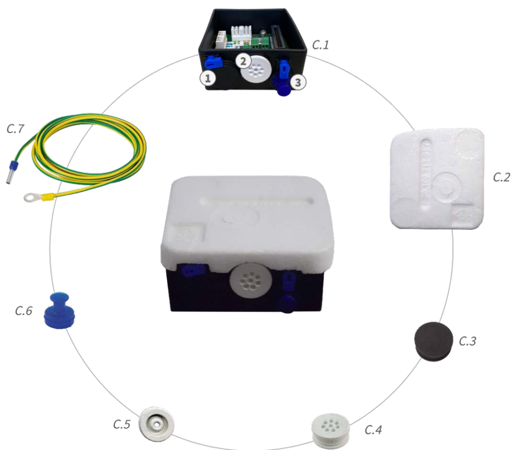
Fig. 2 : Étendue de la livraison MOBOTIX M73 Boîte de connexion LSA
