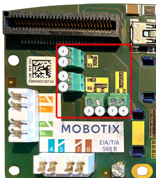
Connettori terminali Scatola di connessione LSA
