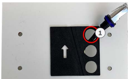
Fig. 10: Preparato per Scatola di connessione RJ45
