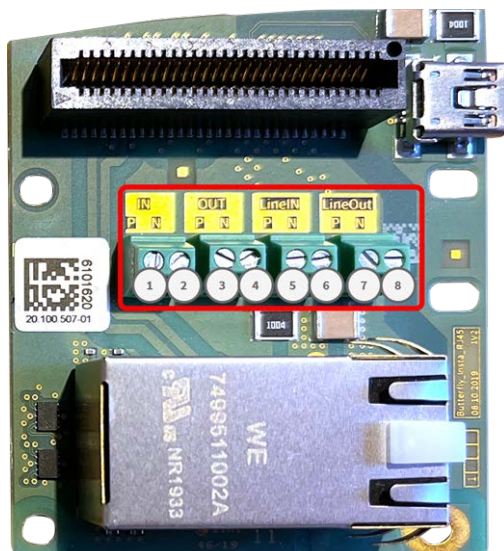
Connettori terminali Scatola di connessione RJ45
