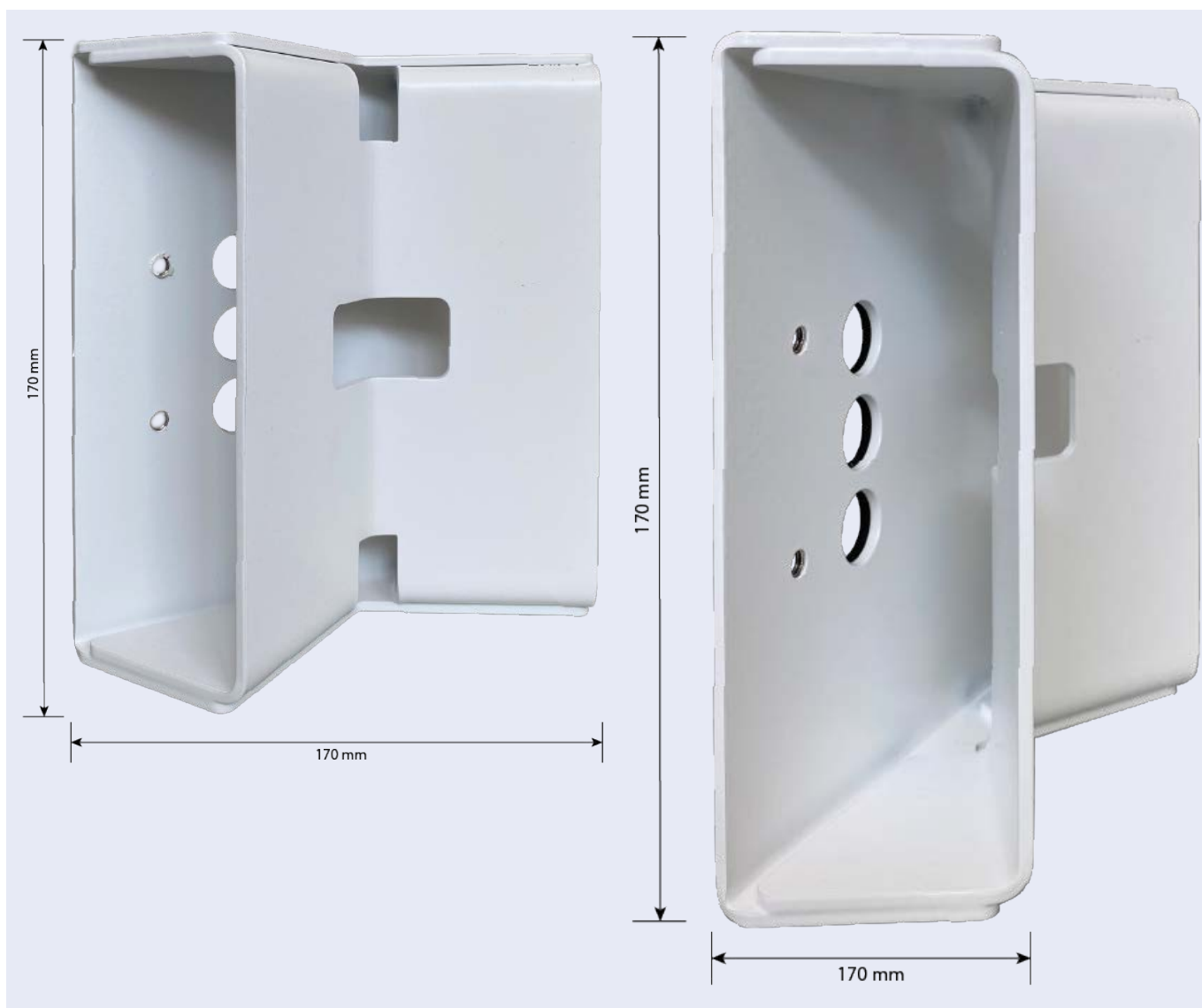
Fig. 8: Dimensioni M73 montaggio su palo - vista posteriore
