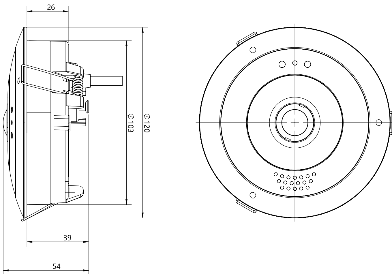
Fig. 1: MOBOTIX c ONE Nurse Assist: Tutte le misure sono espresse in mm
