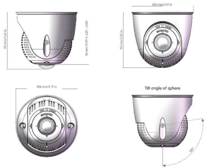
Fig. 2 : PTMount
