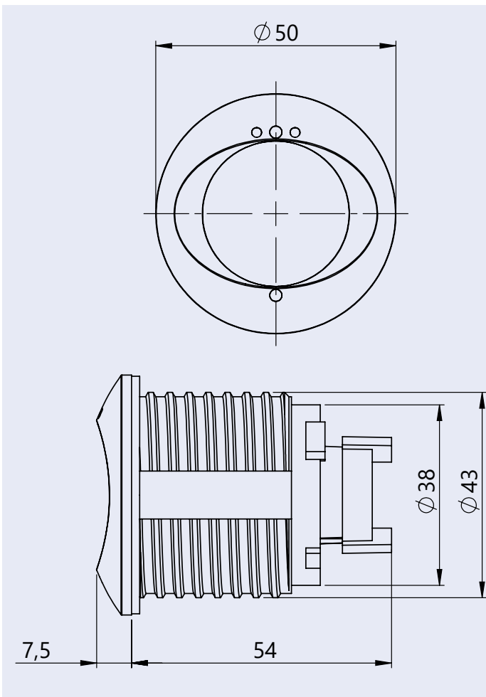
Standard-Sensormodul
