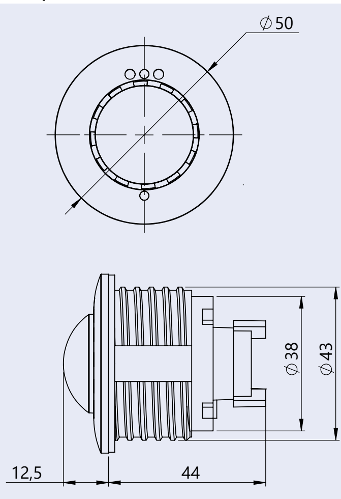
Hemisphärisches Sensormodul
