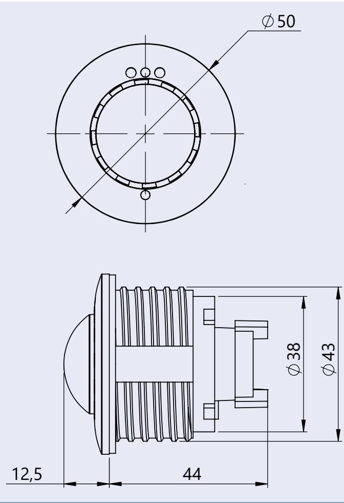
Module de capteur hémisphérique
