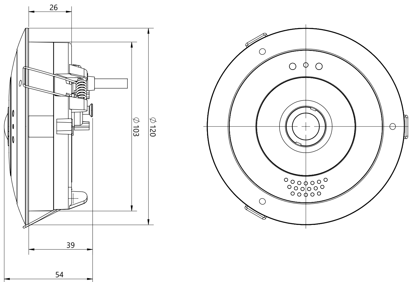
Fig. 1: MOBOTIX c ONE Nurse Assist: Todas las medidas en mm
