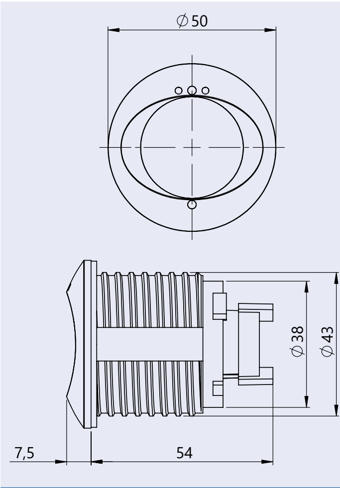
Modulo sensore standard
