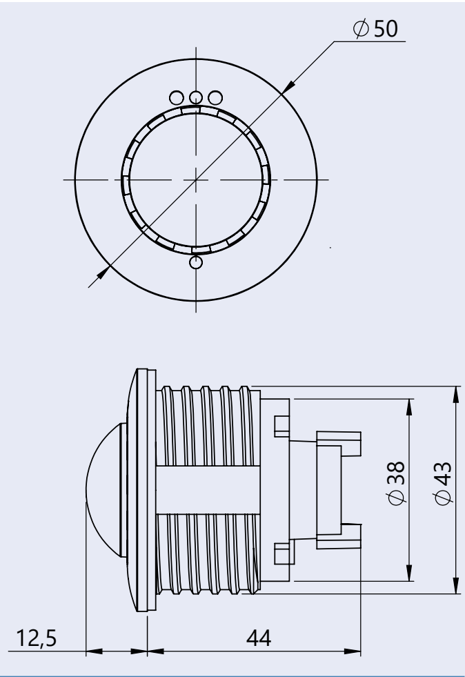
Modulo sensore emisferico
